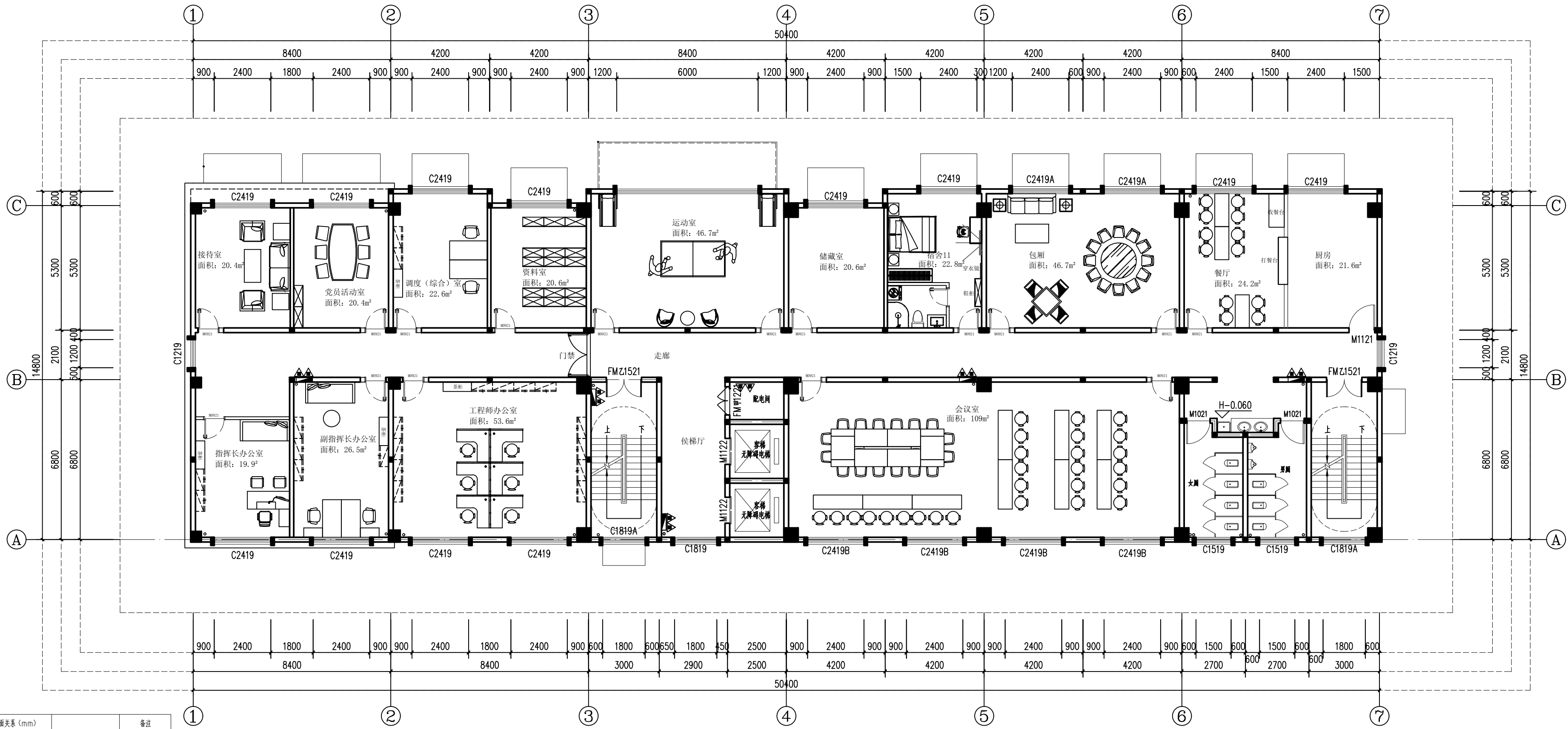
二层平面图 1:100
