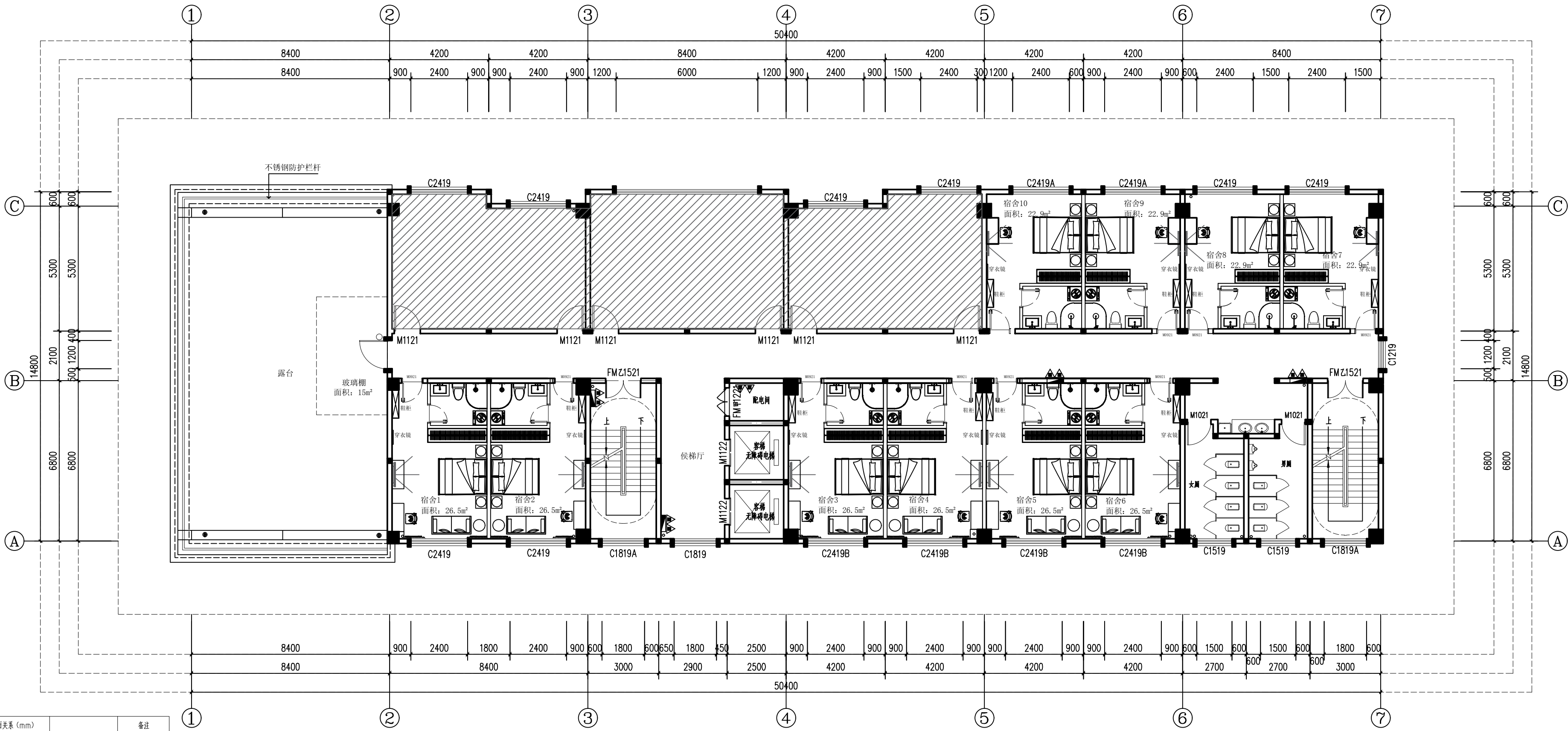
三层平面图 1:100
